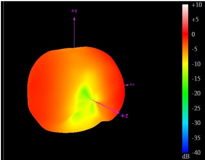
704MHz
