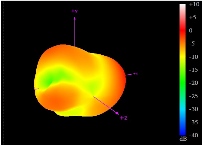
704MHz
