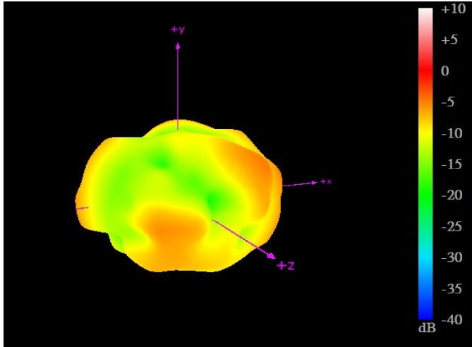
1710MHz
