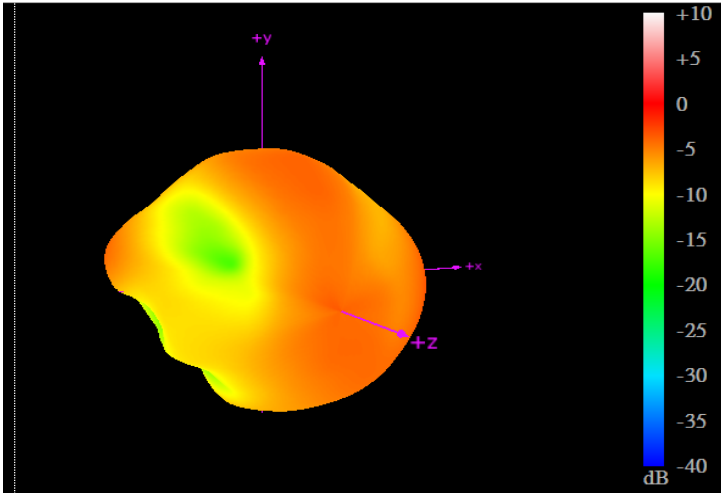
704MHz
