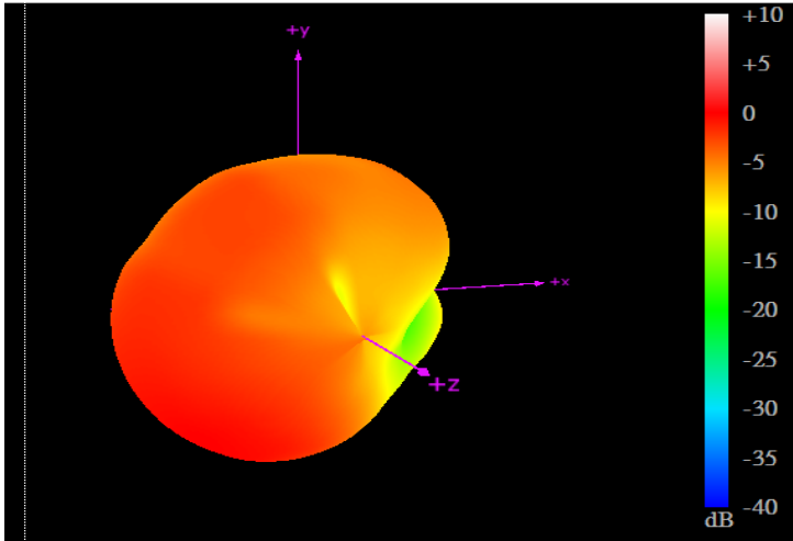
704MHz
