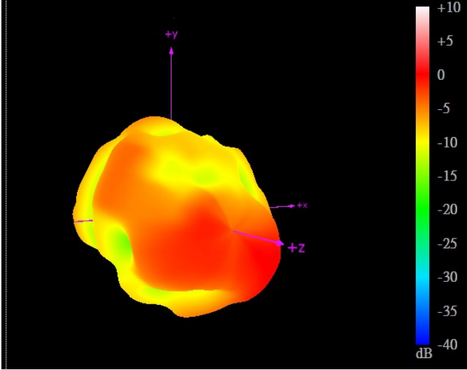
2690MHz
