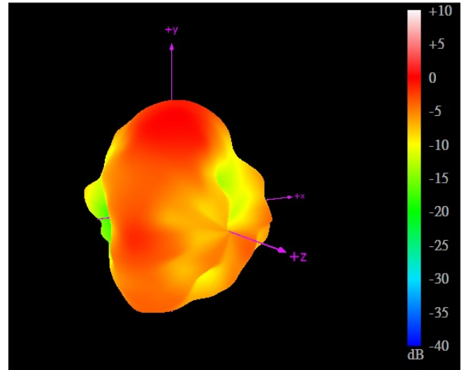
3500MHz
