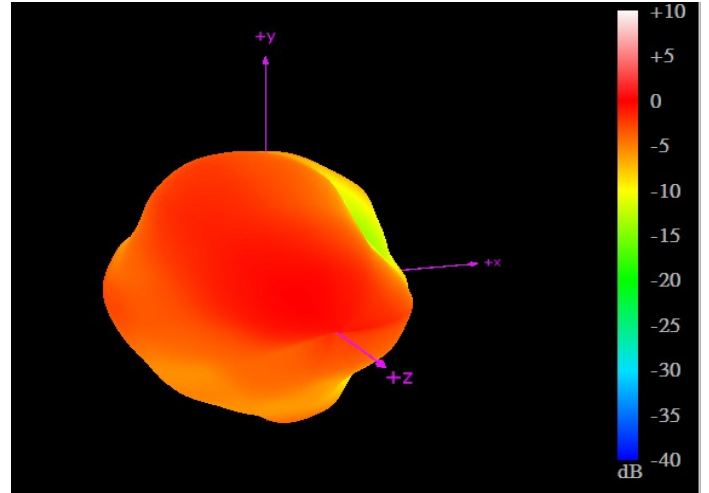
960MHz
