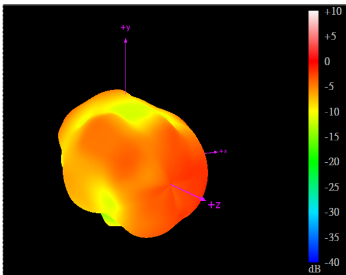
1710MHz
