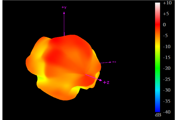
3500MHz
