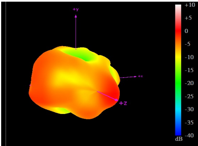
1710MHz
