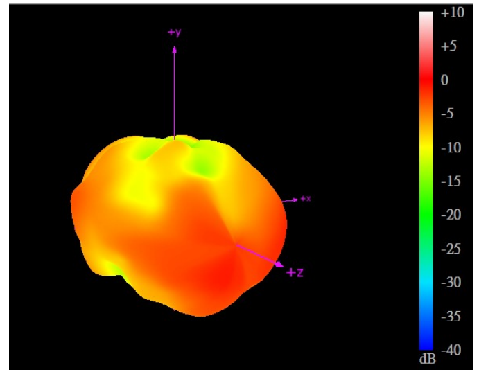
2170MHz
