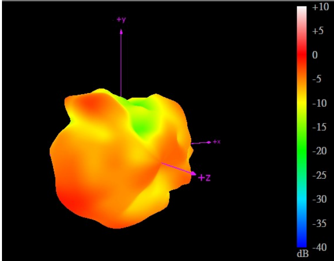
2690MHz
