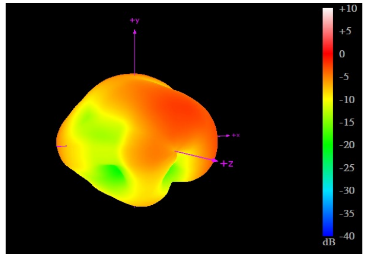
960MHz
