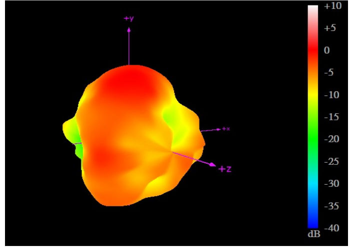
3500MHz
