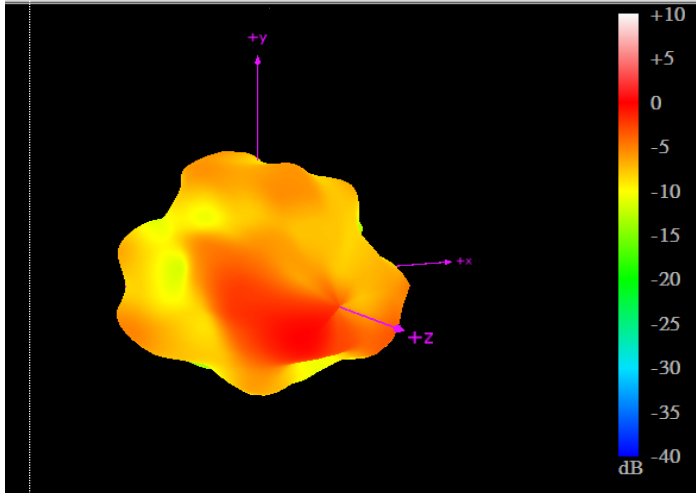
2690MHz
