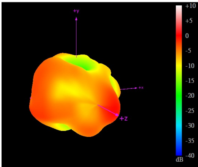
1710MHz
