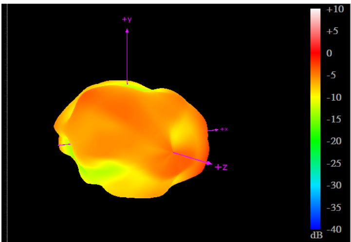
1710MHz
