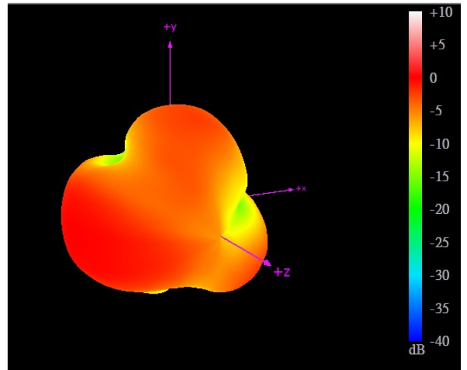
960MHz
