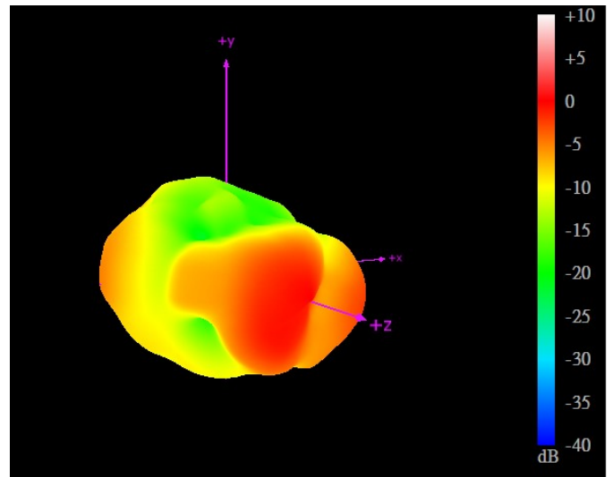
2170MHz
