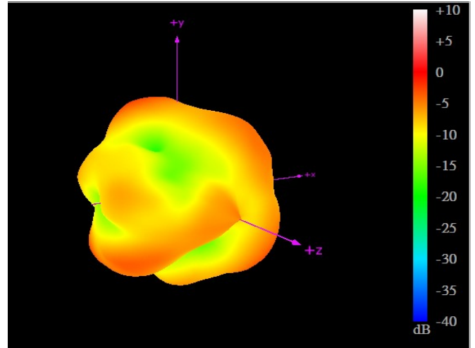
960MHz
