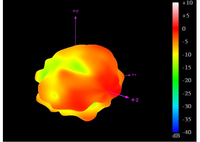
3500MHz
