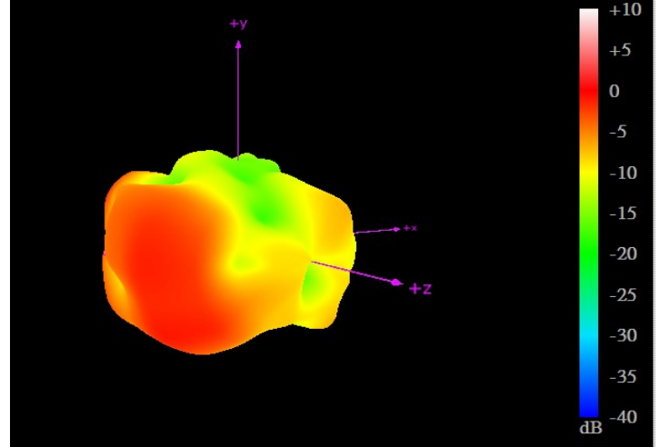
2170MHz
