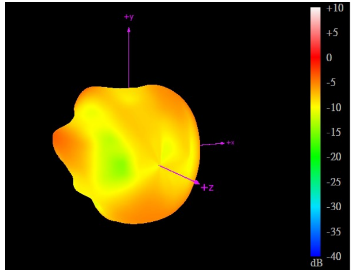
960MHz
