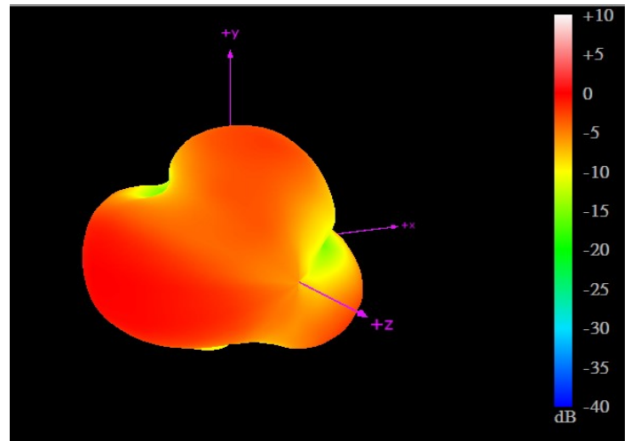
960MHz
