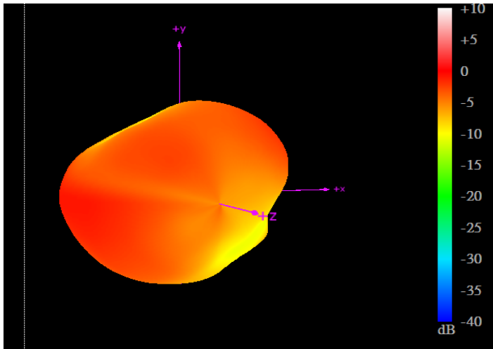
704MHz
