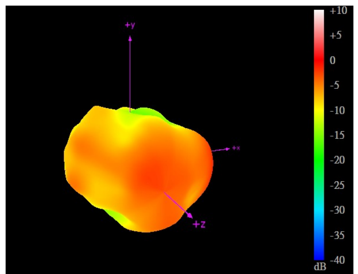
2170MHz
