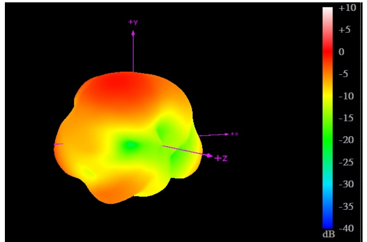
960MHz
