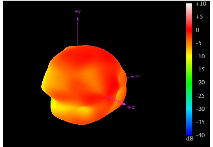
3500MHz
