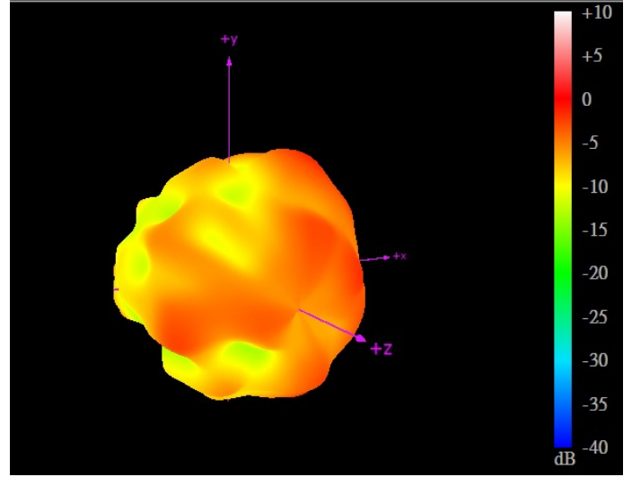
3500MHz
