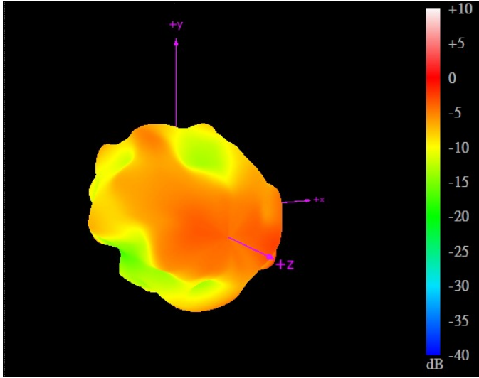
2690MHz
