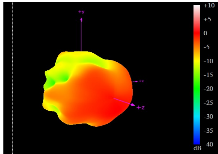
1710MHz
