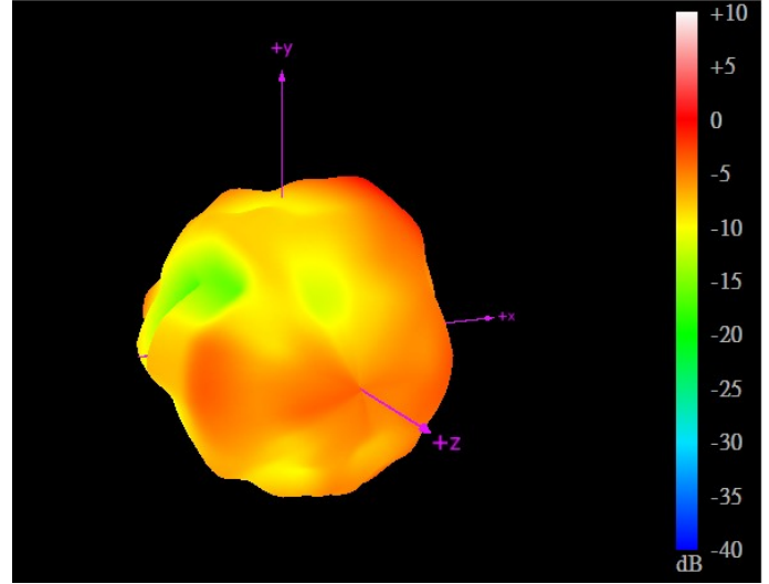
3500MHz
