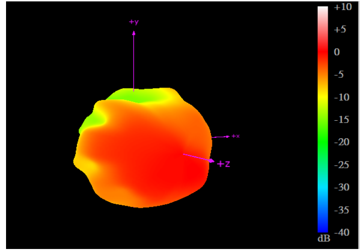
2170MHz
