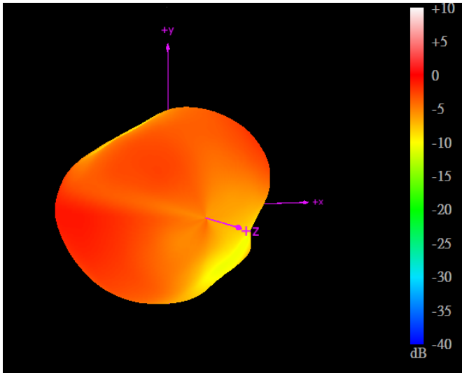
704MHz
