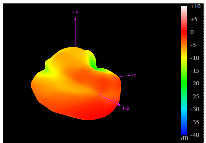
2170MHz
