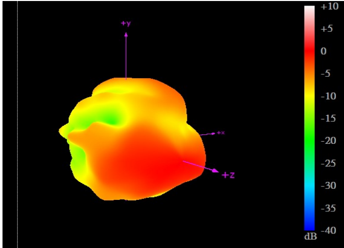
2690MHz
