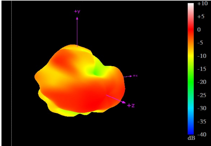
2690MHz
