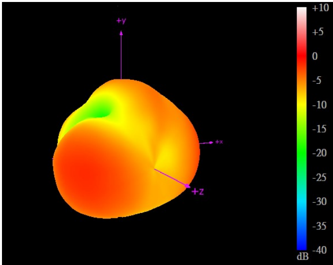
704MHz
