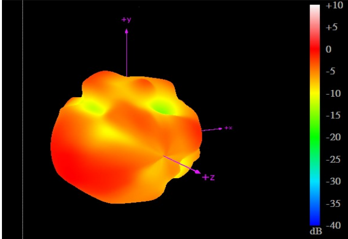
2690MHz
