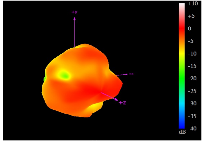
3500MHz
