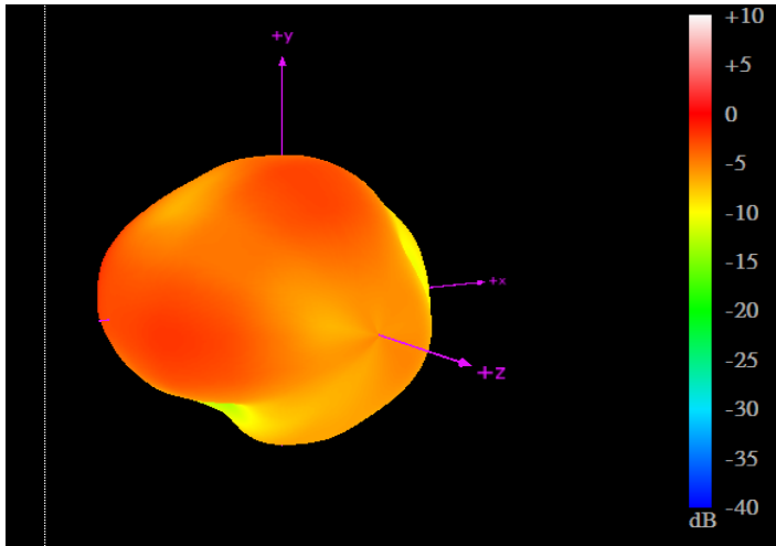
704MHz
