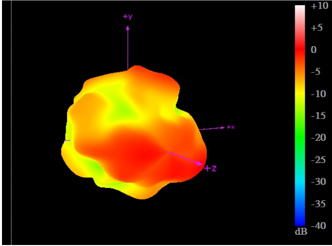
2690MHz
