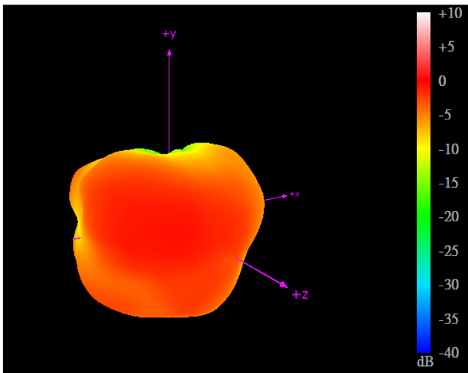
1710MHz
