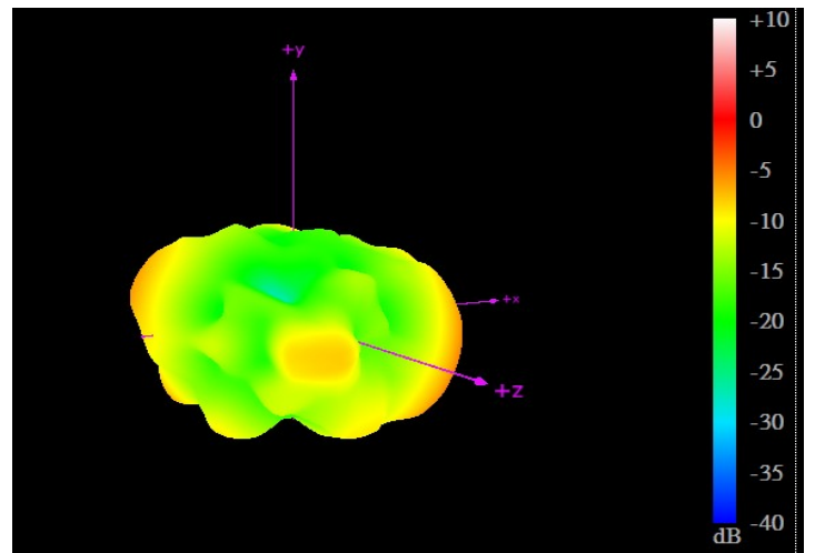
2170MHz
