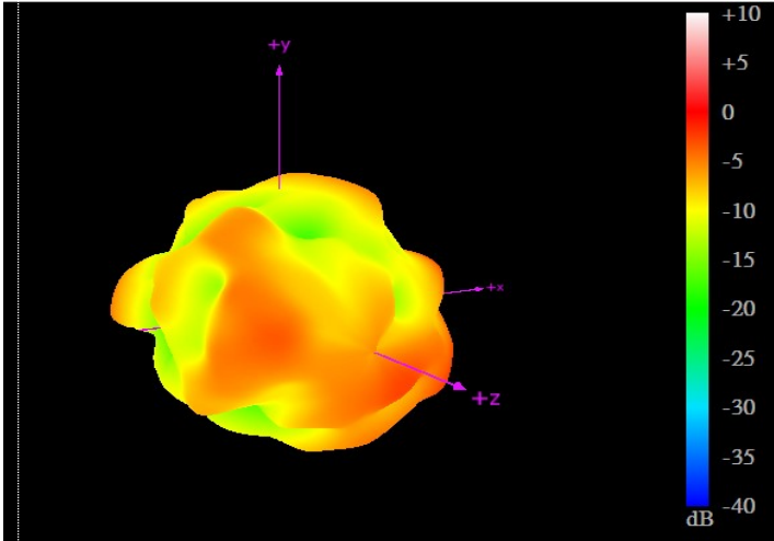
2690MHz
