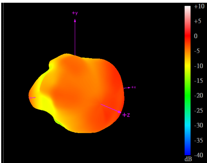
1710MHz
