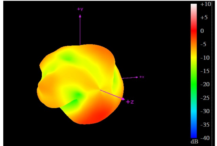
960MHz
