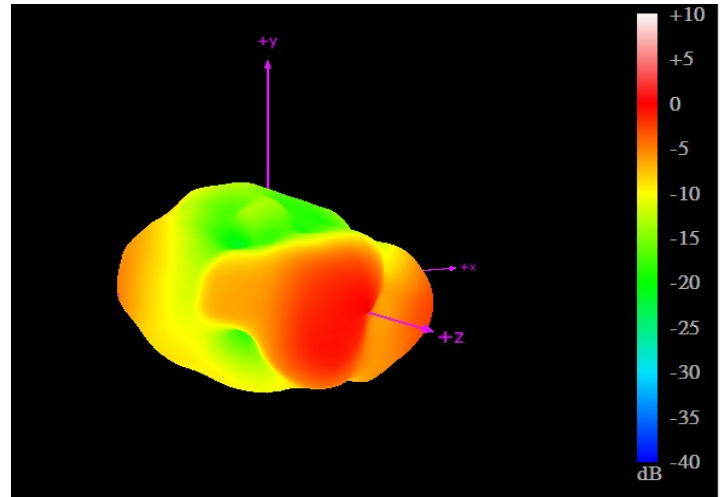
2170MHz
