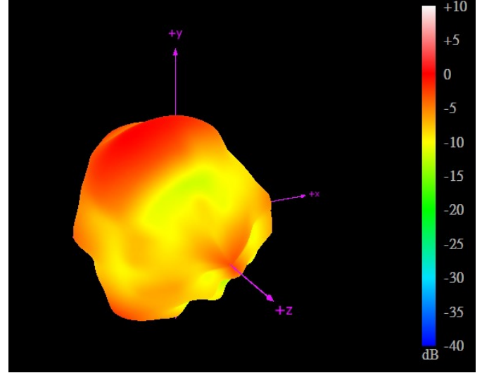
3500MHz
