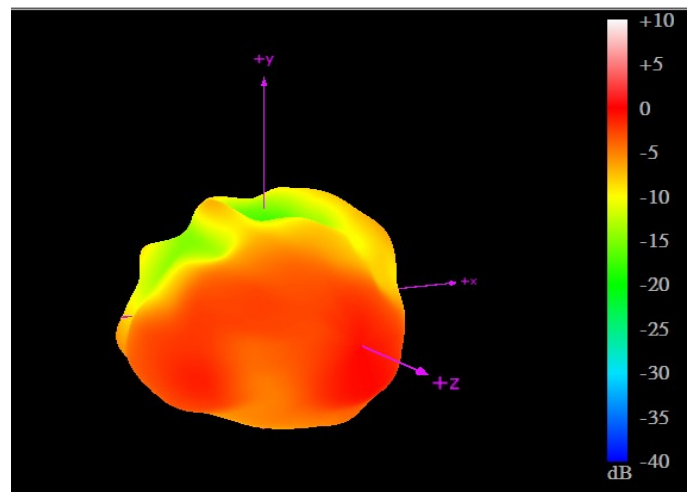
2170MHz
