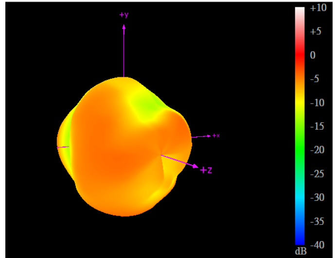
960MHz
